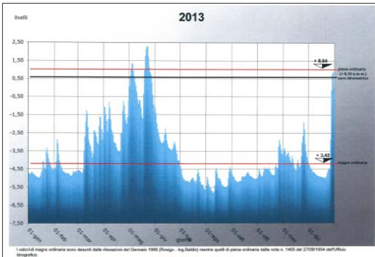
Graf. 1.39 - Livelli idrometrici giornalieri del fiume Po (m. rispetto allo zero idrometrico), rilevati alle ore 8.00 presso l'idrometro di Pontelagoscuro per l'anno 2013
