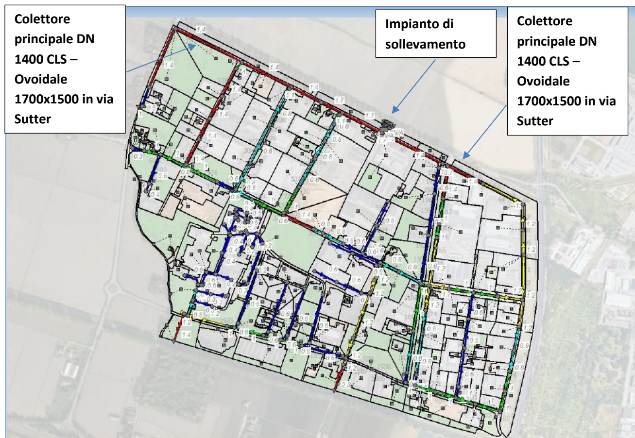
Fig. 18 – Estratto della cartografia delle reti fognarie rilevate – zona nord
