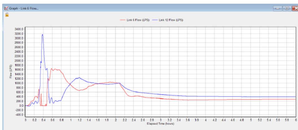
Fig. 52 – Portata nei rami terminali di via Sutter a monte dell'impianto di sollevamento
