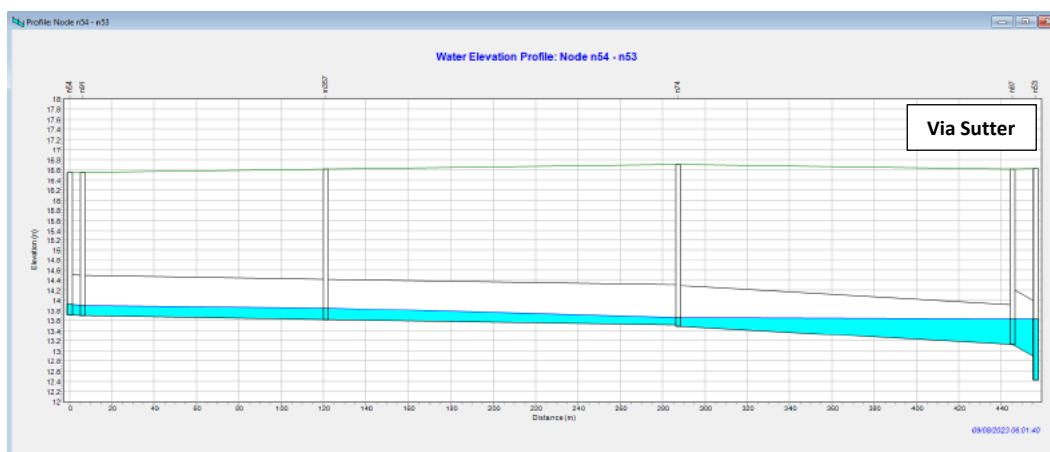
Fig. 34 – Profilo collettore principale via Gessi (pendenza da via Finati verso via Sutter)
