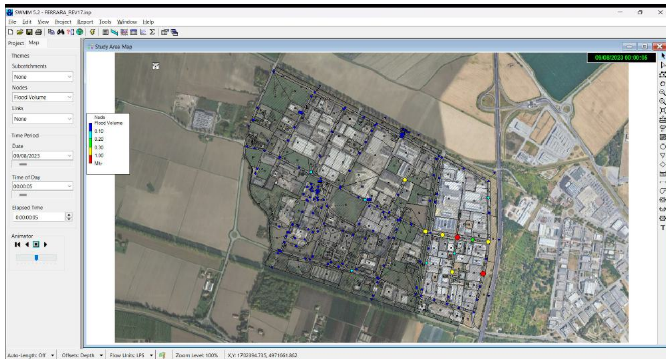
Fig. 55 – Nodi idraulici nei quali si potrebbe verificare il fenomeno del “flooding”
